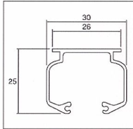
ハンガーレールの形状
