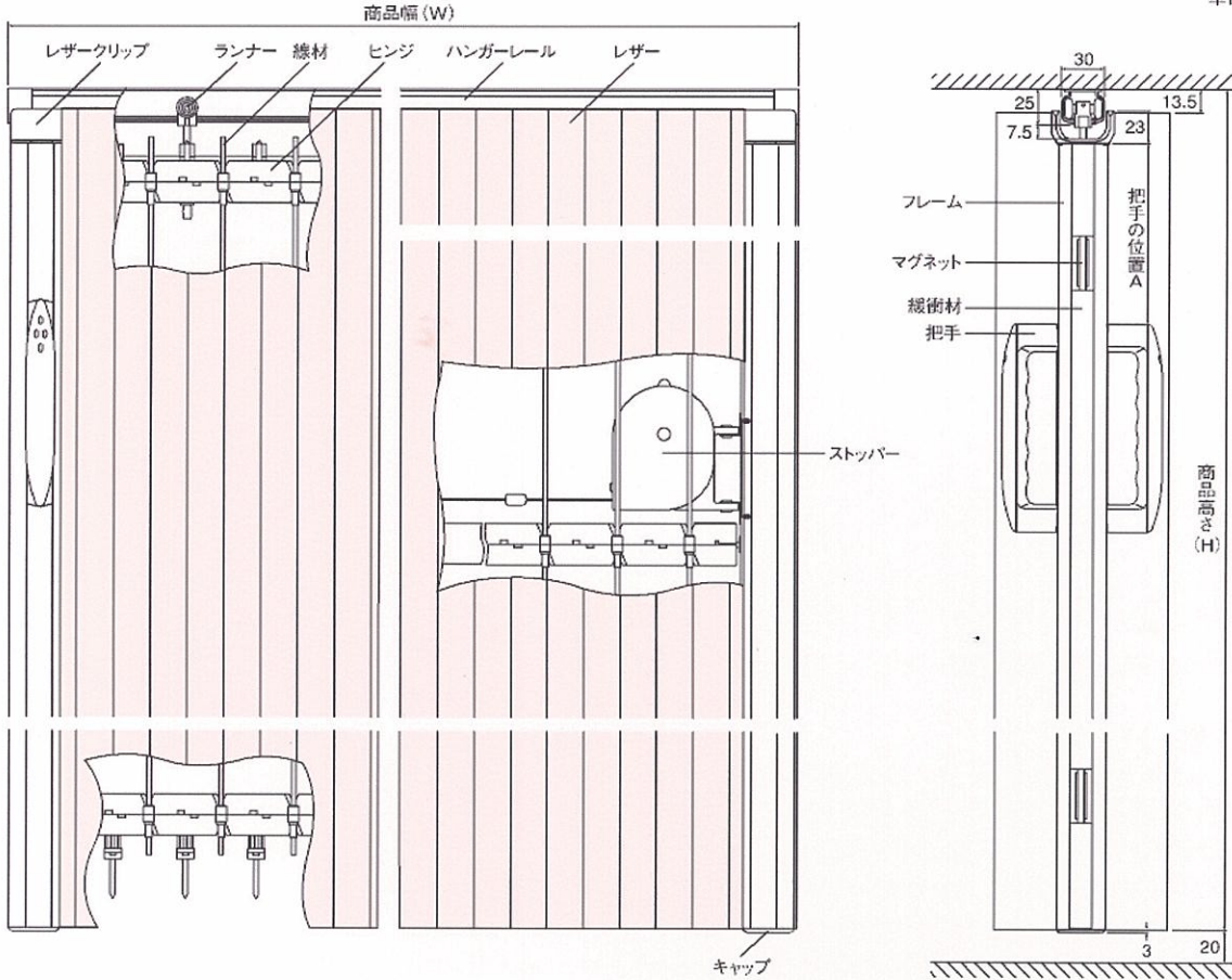
ハンガーレールの形状
